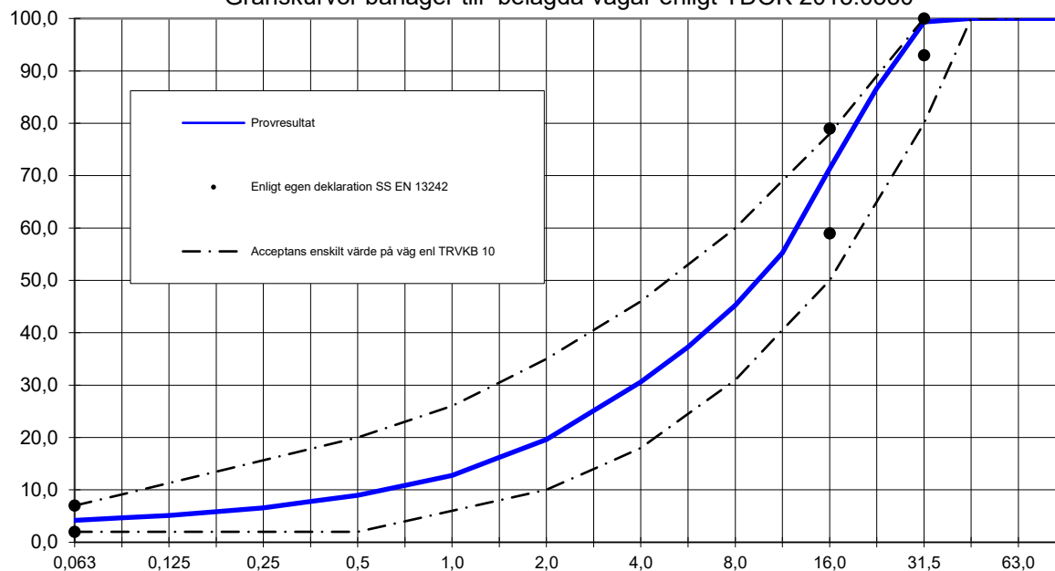
Gränskurvor bärlager till belagda vägar enligt TDOK 2013:0530
