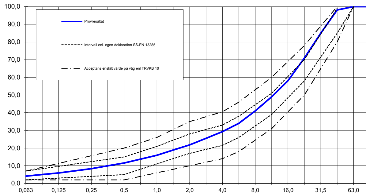
Gränskurvor bärlager till belagda vägar enligt TRVKB 10 2011:083
