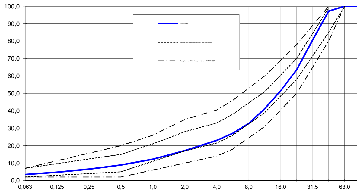
Gränskurvor bärlager till belagda vägar enligt VVTBT 2007:117
