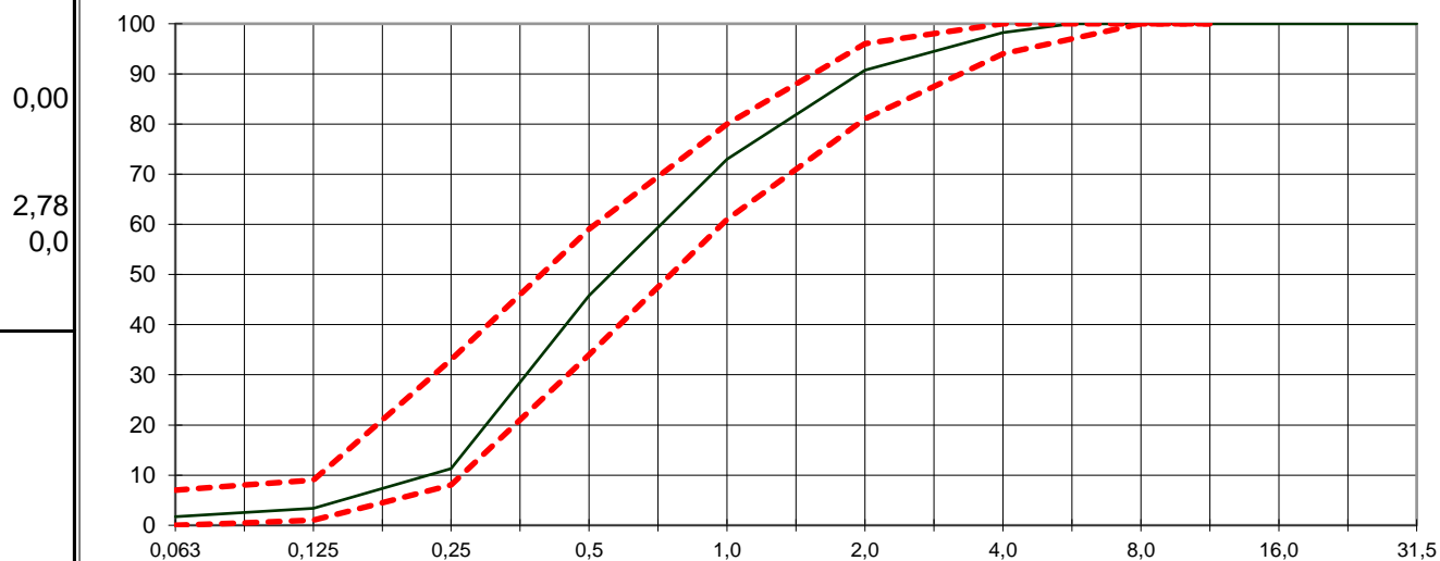
Begränsningslinjer enl. Anl. AMA (Tabell DCJ 12.1)
