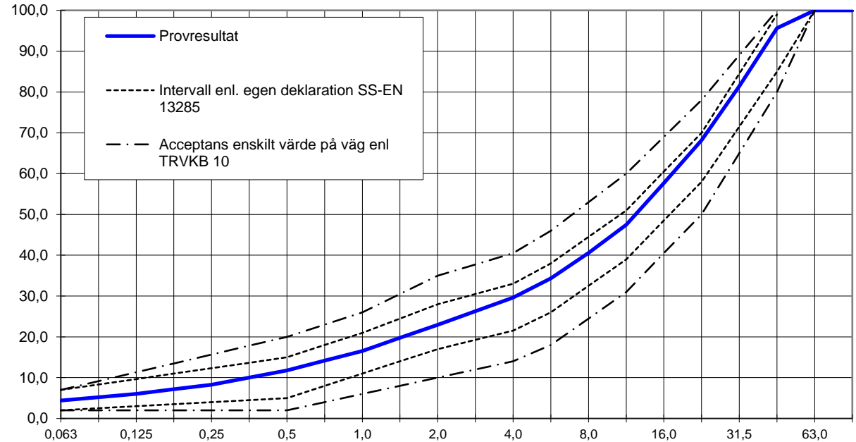
Gränskurvor bärlager till belagda vägar enligt TRVKB 10 2011:083
